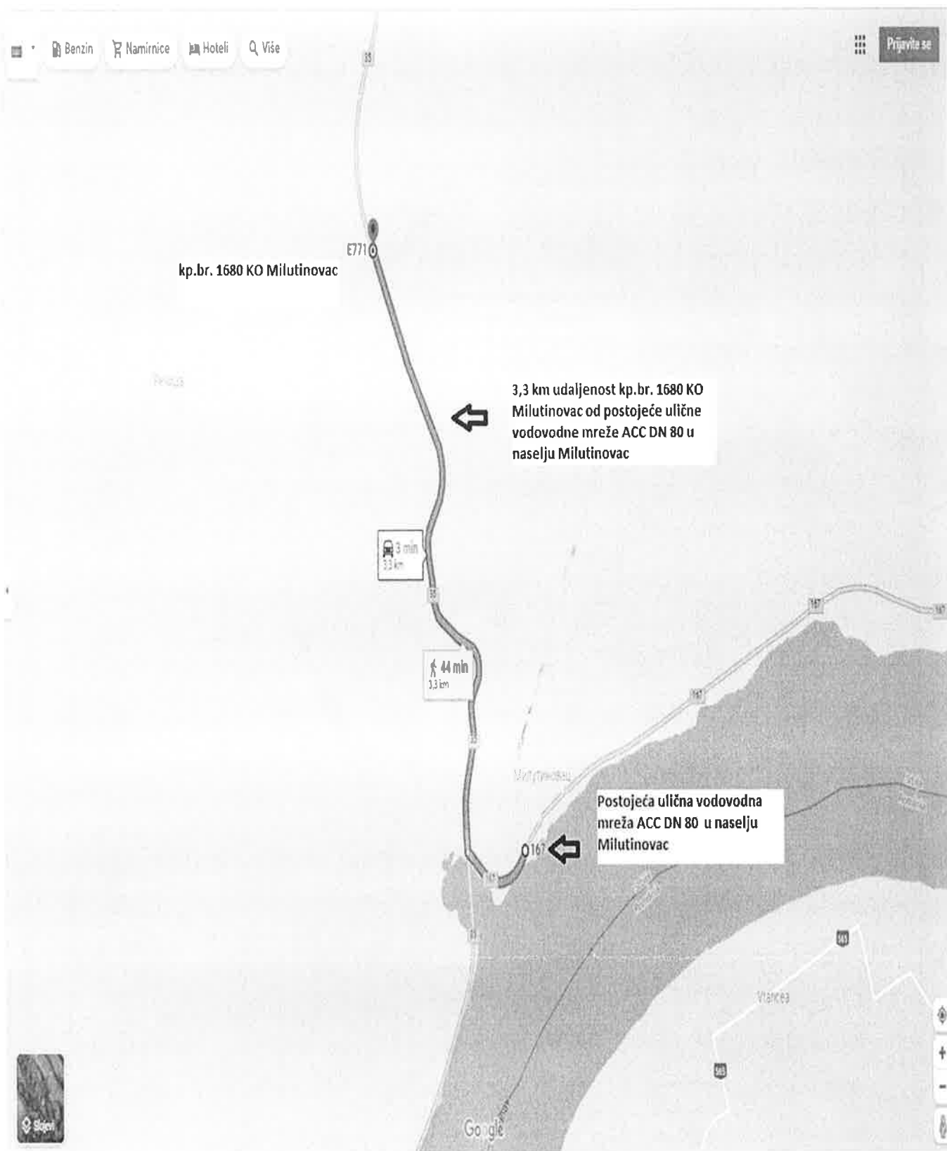
Удаљеност кп.бр. 1680 КО Милутиновац од постојеће уличне водоводне мреже ACC DN 80 у насељу Милутиновац
