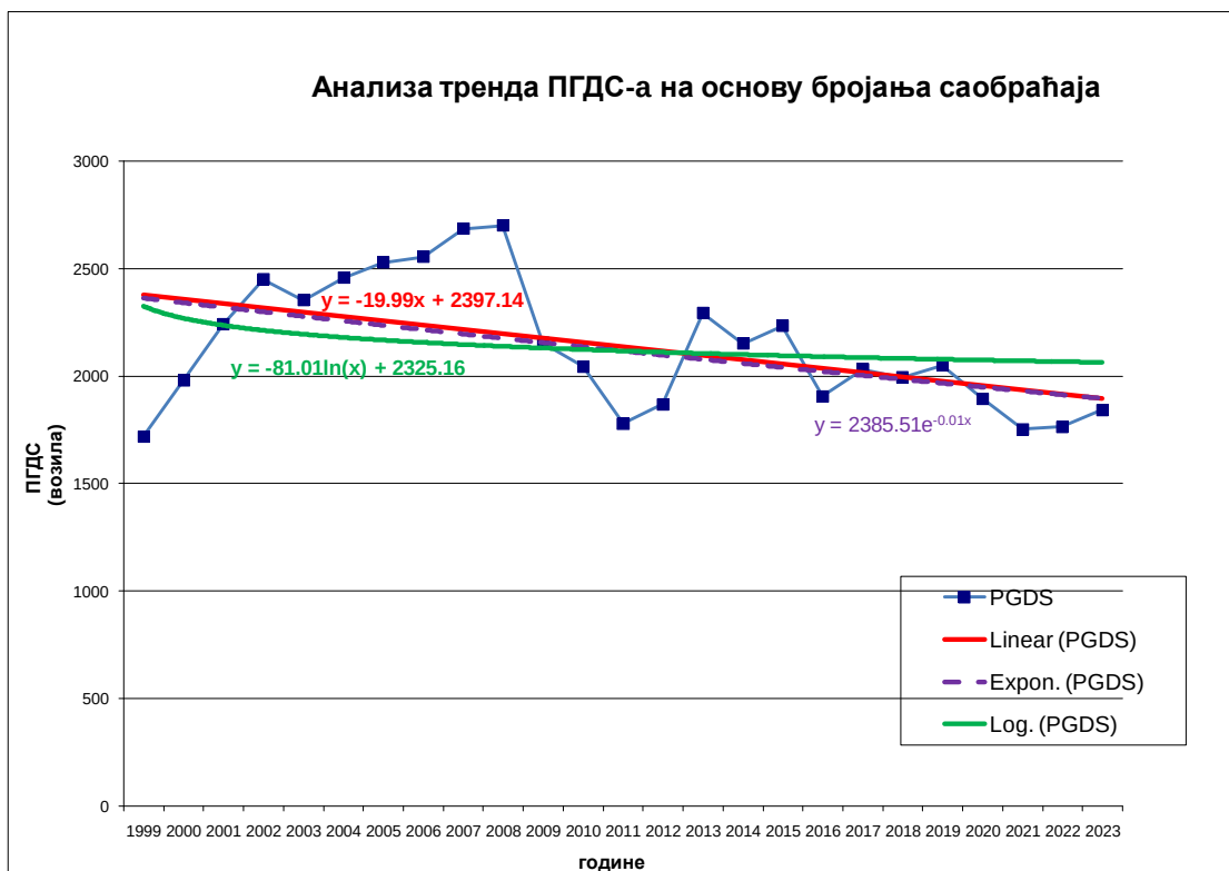
Слика 2 – Анализа тренда саобраћајног оптерећења деонице Кладово-Милутиновац
